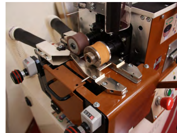
Rulli accoppiatura - Combining rollers
